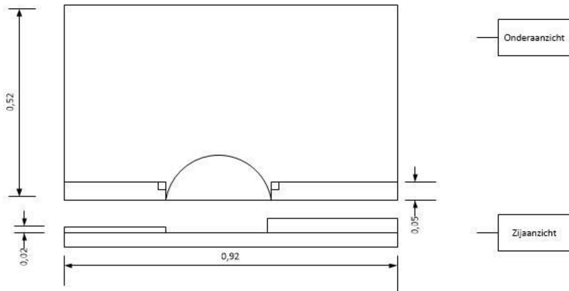
Afb. 10 Tekening hulpstuk
