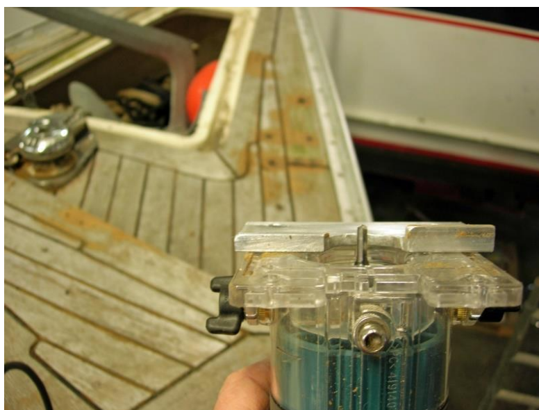
Afb. 9 Freesmachine (op de kop) met frees en gemonteerd hulpstuk
