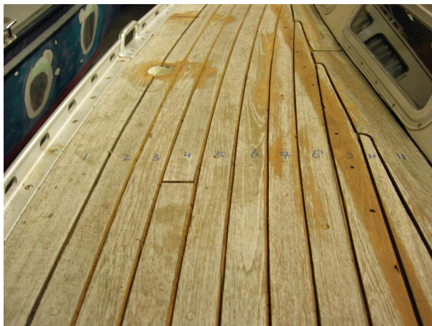
Afb. 14 Groeven gefreesd
