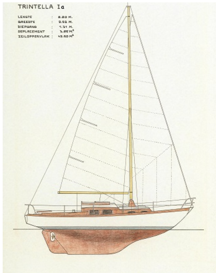
Voorbeeld van een profieltekening van een Trintella la
